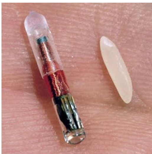
Figure 18 : Une puce RFID à côté d'un grain de riz.
