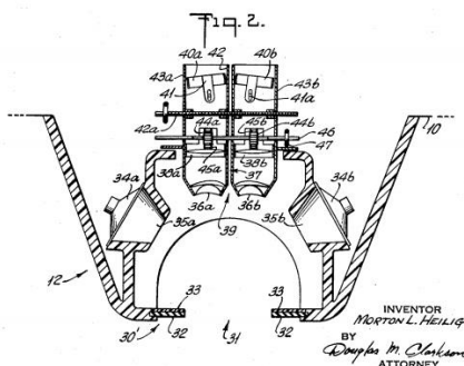
Figure 7 : Diagramme de Fonctionnement du Sensorama de Morton L. Heilig pour le bureau des brevets américains 4 . L'utilisateur place sa tête en face des deux objectifs en bas.
